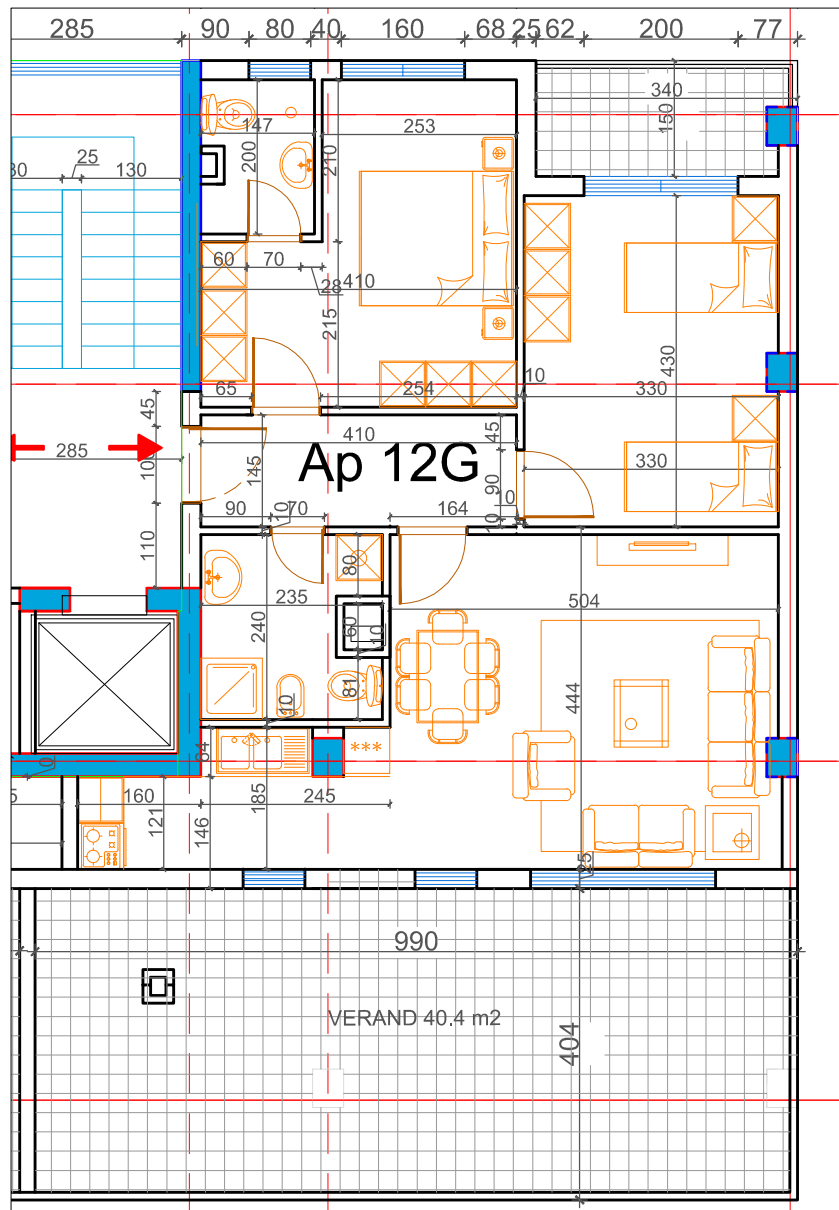
PLANIMETRIA E APARTAMENTIT (mobilim dhe dimensionim) shkalle_1:100
